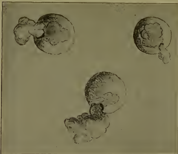
Fig. 160. Lachseier, deren Inhalt ausläuft.
